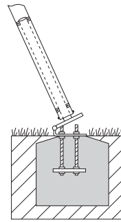
Kipphalterung aus Stahl mit Sicherheitscharnier und Justierbolzen
